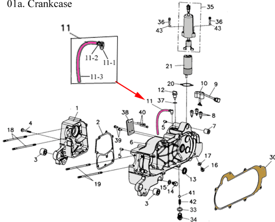
01a. Crankcase
